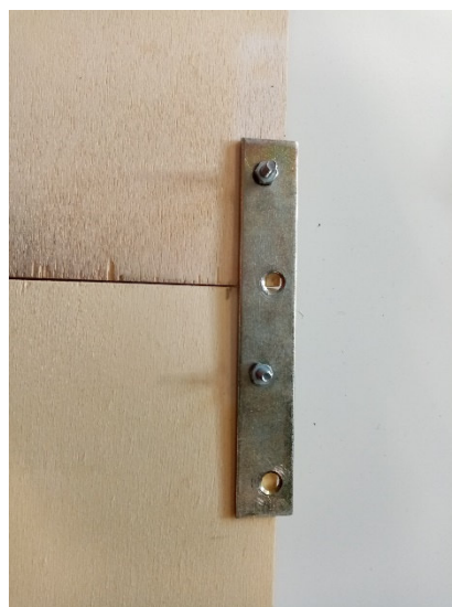
Eine Möglichkeit, zwei Sperrholzplatten miteinander zu verbinden, falls die Rennbahn länger werden soll
